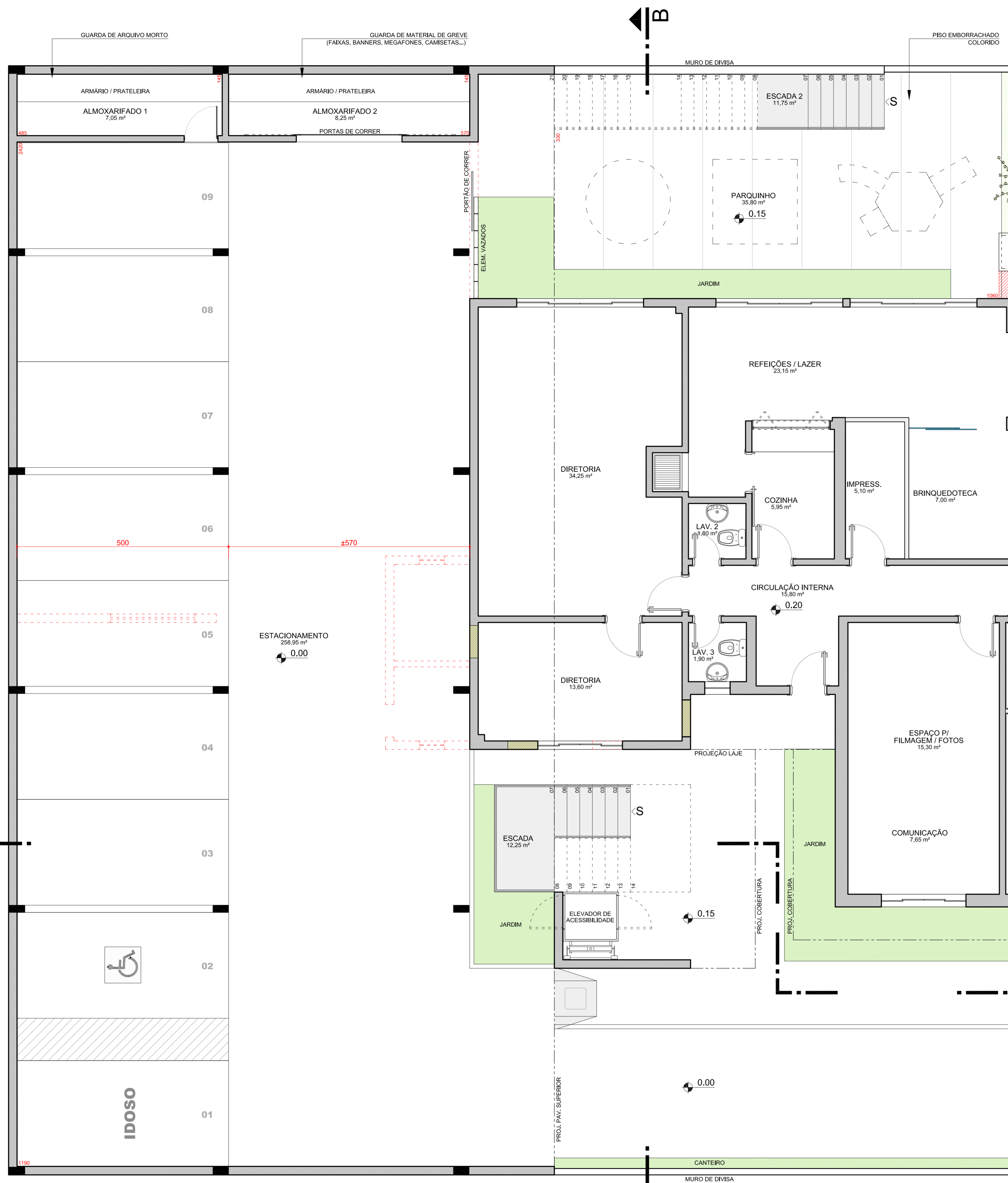
PLANTA PAV. TÉRREO ESCALA 1:50 ÁREA COMPUTÁVEL: 594,10 m² ÁREA NÃO COMPUTÁVEL: 3,25 m² ÁREA TOTAL: 597,35 m²
