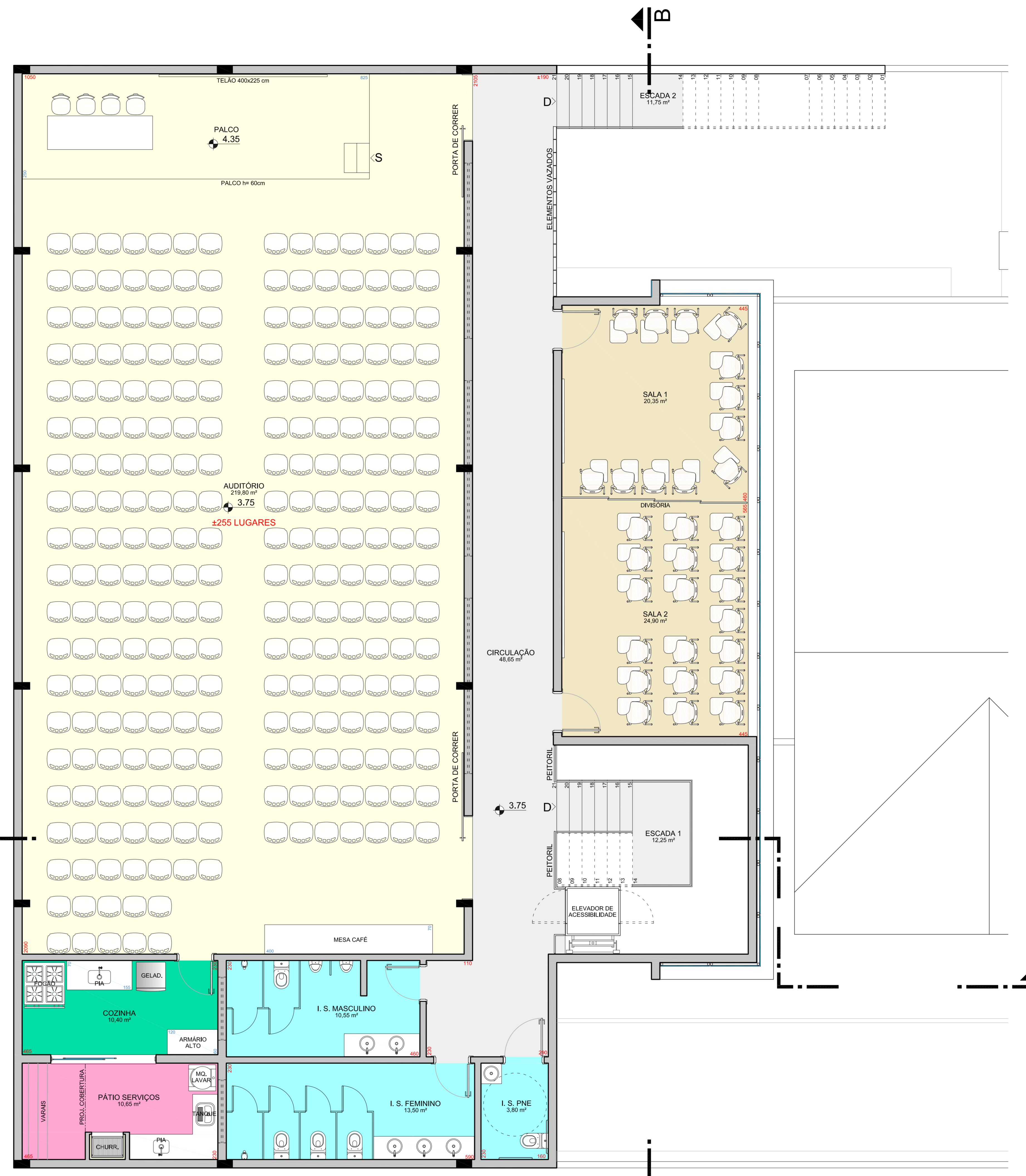
PLANTA PAV. SUPERIOR ESCALA 1:50 ÁREA COMPUTÁVEL: 397,00 m² ÁREA NÃO COMPUTÁVEL: 3,25 m² ÁREA TOTAL: 400,25 m²
